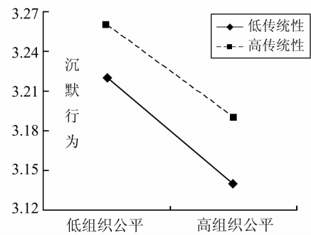
图 2 调节效应图
